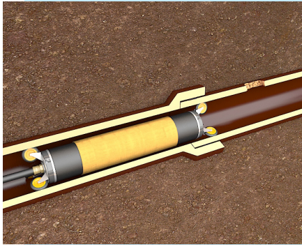
(a) Reparatur mit Kurzlinern Positionierung des Packers mit dem Kurzliner
