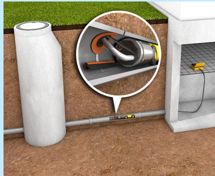
Roboterverfahren z.B. Injektion, Verpressen, Verspach- teln (nur bedingt einsetzbar, da i.d.R. erst ab DN 200 möglich)
