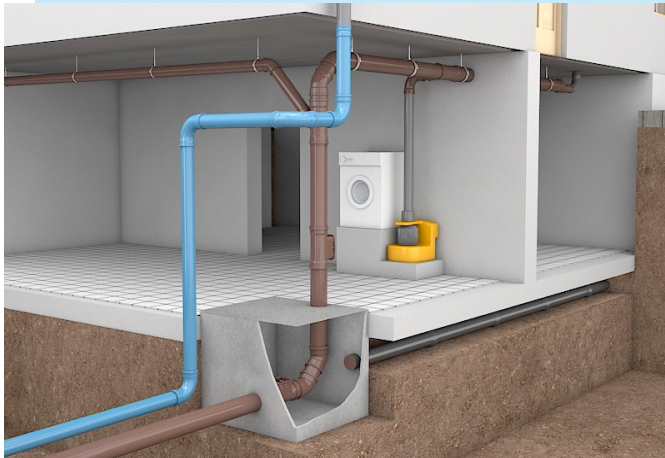
Abhängen neuer Leitungen im Kellerbereich
