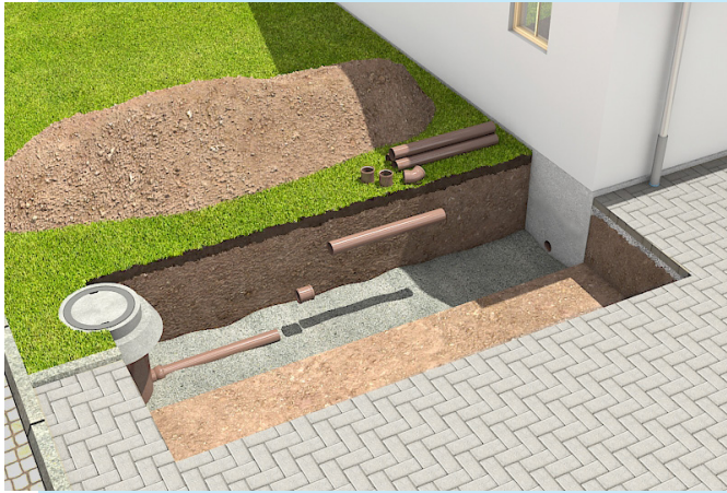
Erneuerung in offener Bauweise
