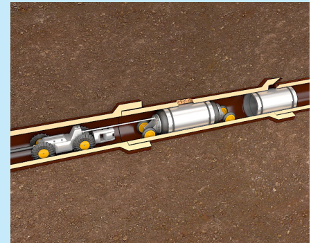
Innenmanschetten Positionierung der Manschette mit dem Kamerawagen (nur bedingt ein- setzbar, da nur sehr eingeschränkt bogengängig)
