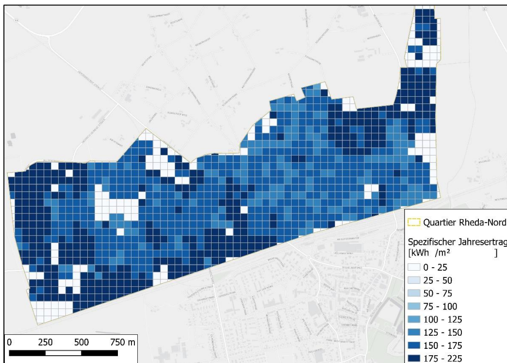
Abbildung 43 | Potenzialabschätzung des spezifischen Jahresstromertrags von Dach-PV-Anlagen basierend auf den Ausrichtungen und den Neigungswinkeln der Dachflächen (Datenquelle: [LANUV; 2023], eigene Darstellung)
