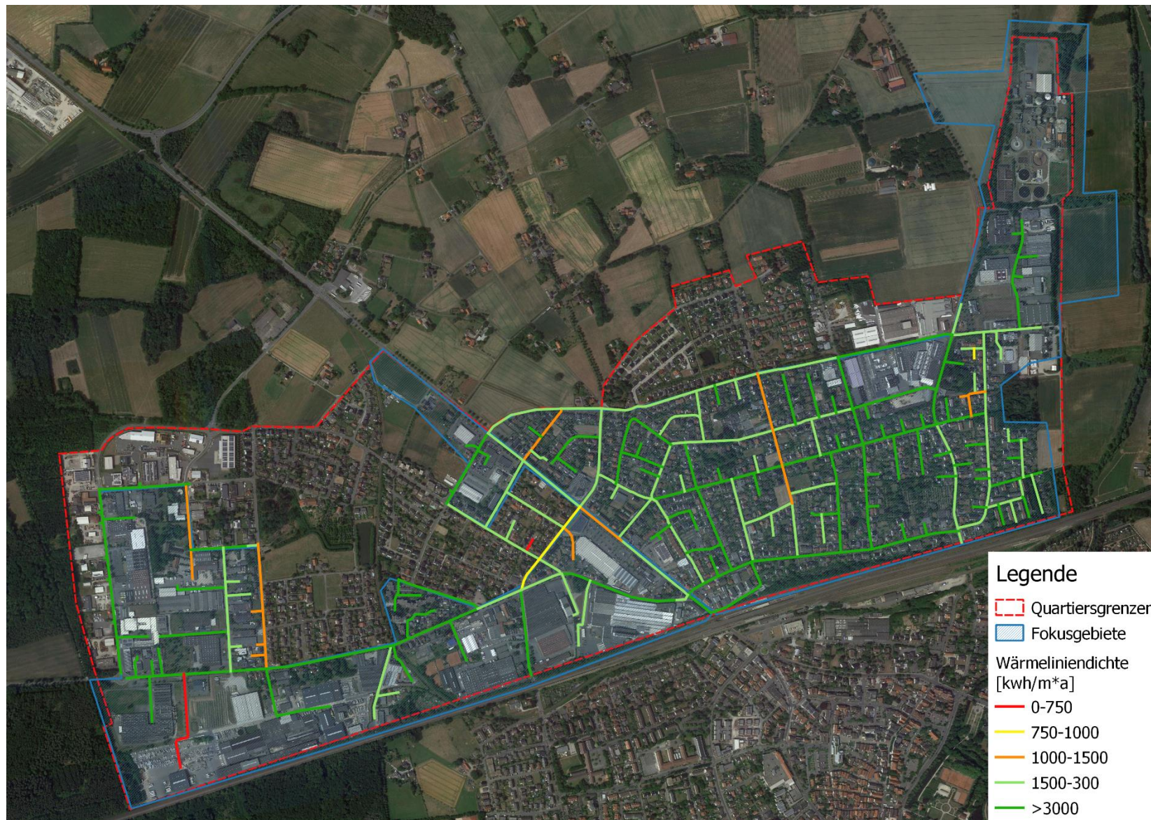
Abbildung 50 | Wärmelinien-dichte und Wirtschaftlichkeit eines theoretischen Wärmenetzes im Quartier Rheda-Nord
