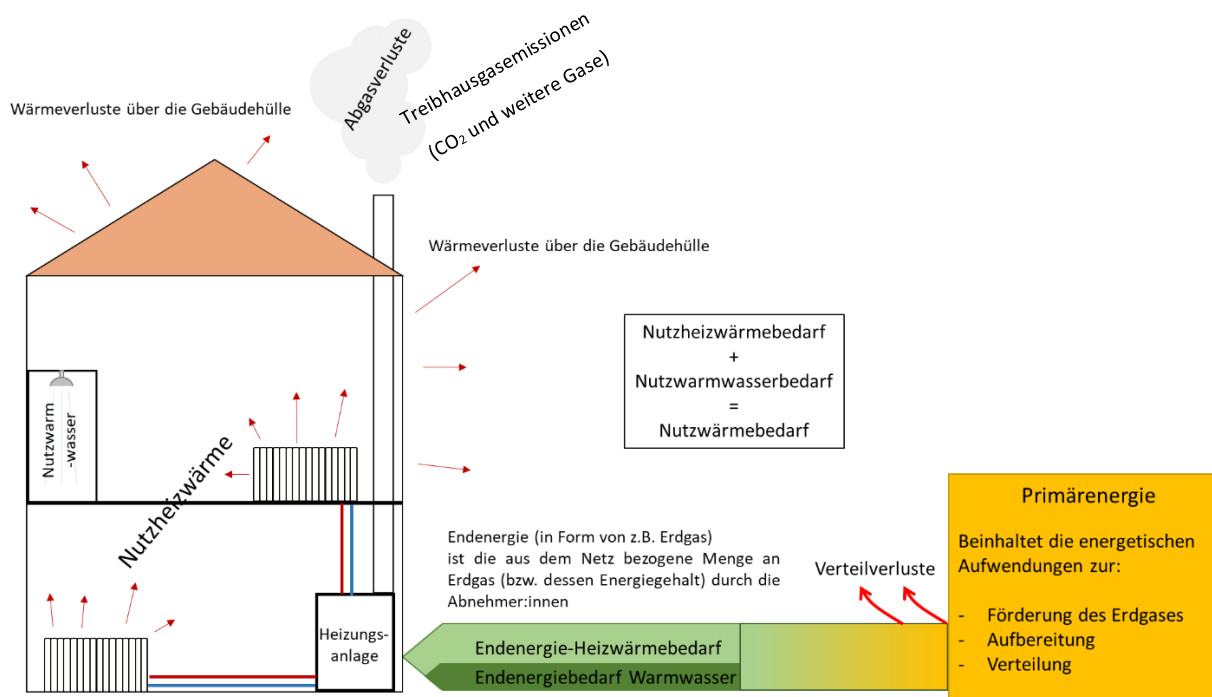
Abbildung 22 | Grafische Erläuterung einiger Energiewirtschaftlicher Fachbegriffe am Beispiel der Gebäudebeheizung mittels des (leitungsgebundenen) Energieträgers Erdgas
