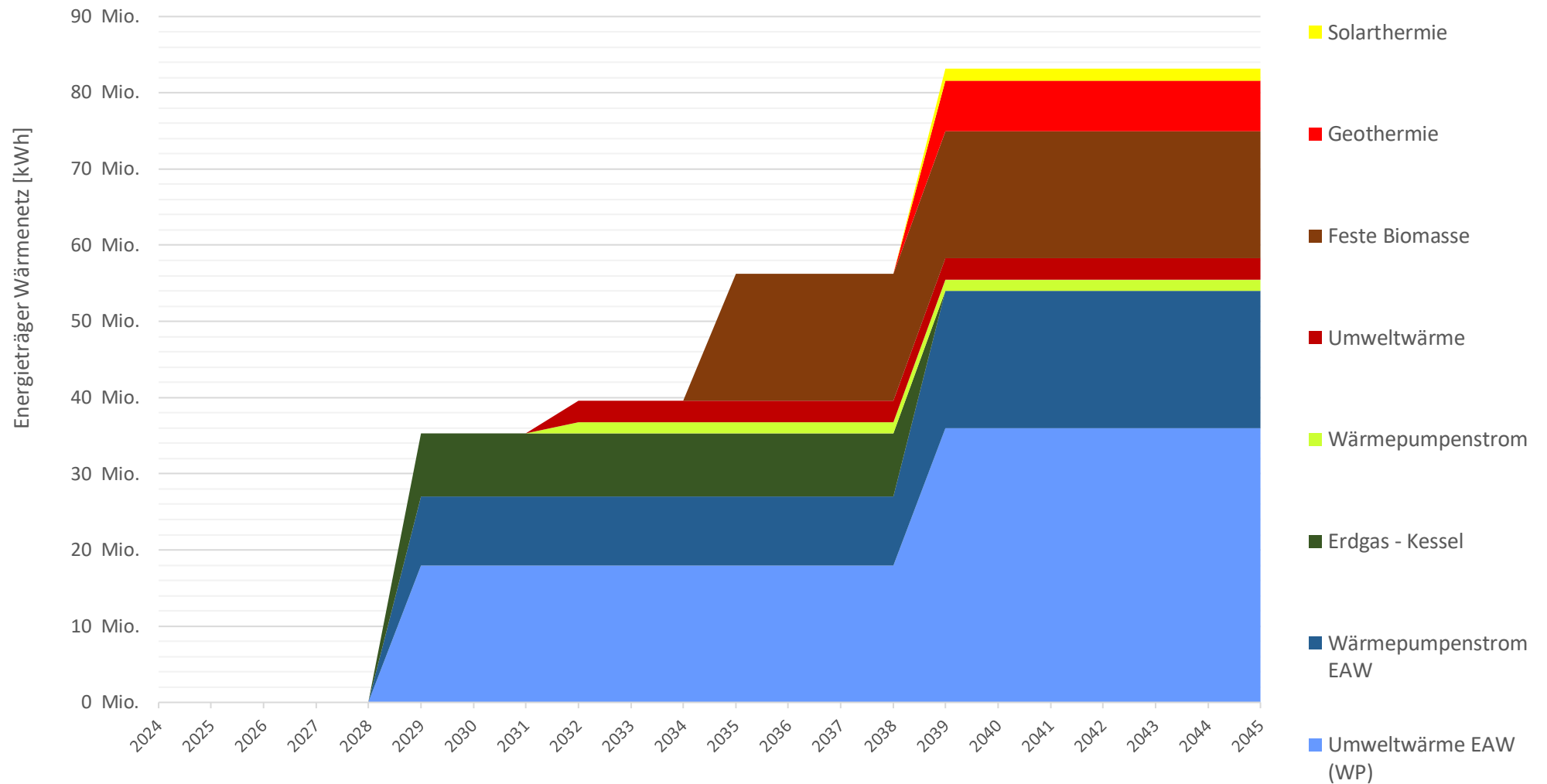
Abbildung 54 | Entwicklung der Energieträgeranteile zur Deckung des Wärmebedarfes eines Wärmenetzes – Szenario 2.1
