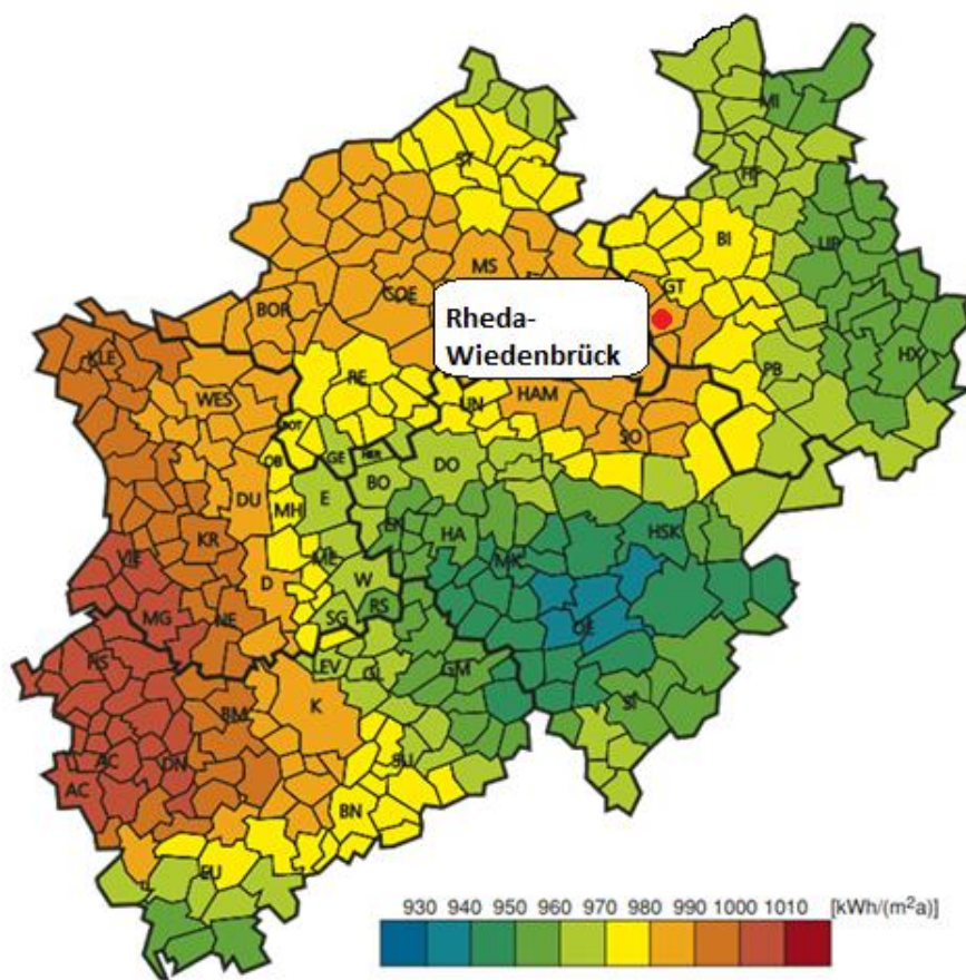
Abbildung 41 | Jahresdurchschnittliche Globalstrahlung Nordrhein-Westfalen (Quelle: [EA NRW])
